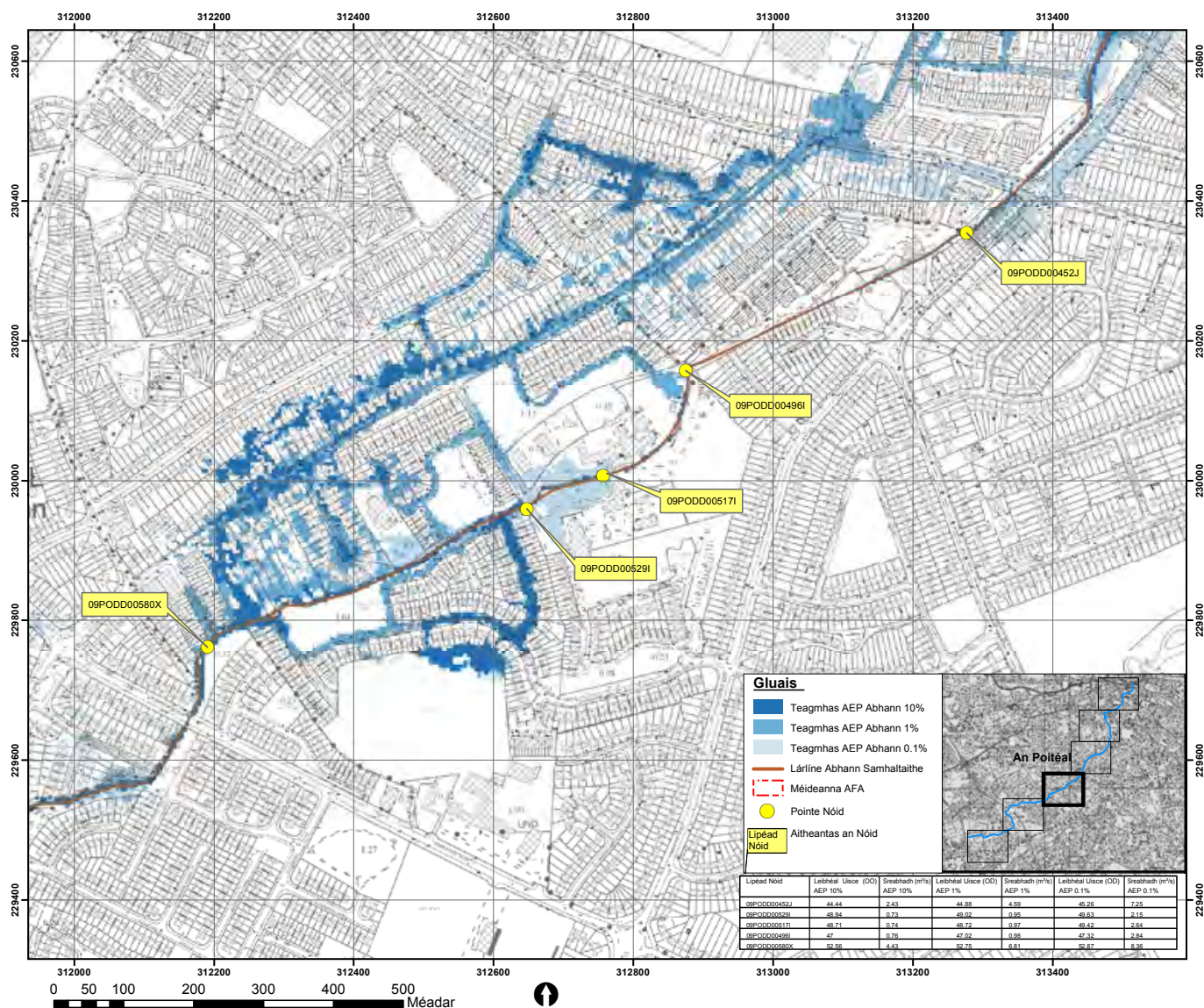
Fíor 8 Méideanna Tuile Abhann an Phoitéil (Foinse: Arna oiriúnu ón Taifead ar Dhéanmhais Chosanta/Oifig na nOibreacha Poiblí)
