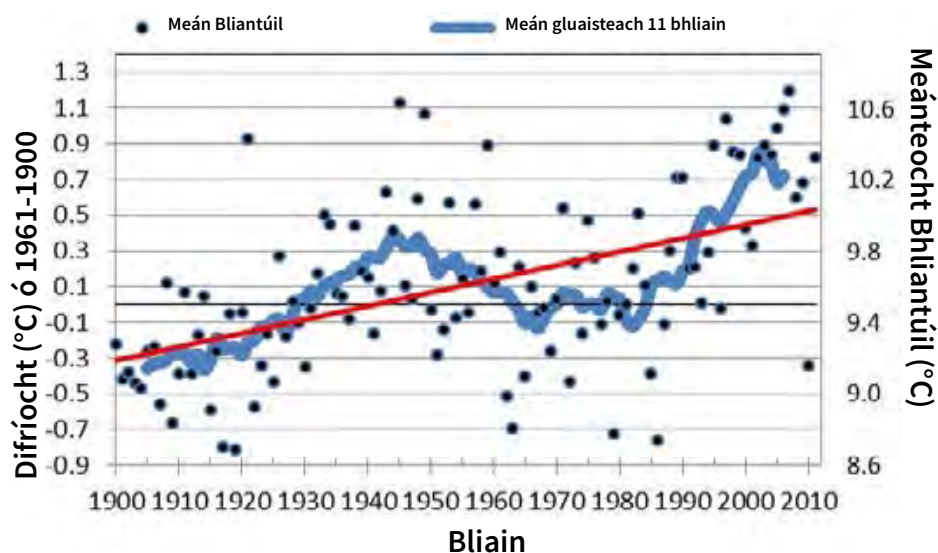
Fíor 6 Meánteocht Aeir Dromchla (1900-2011) (Foinse: An GCC / Dwyer)
